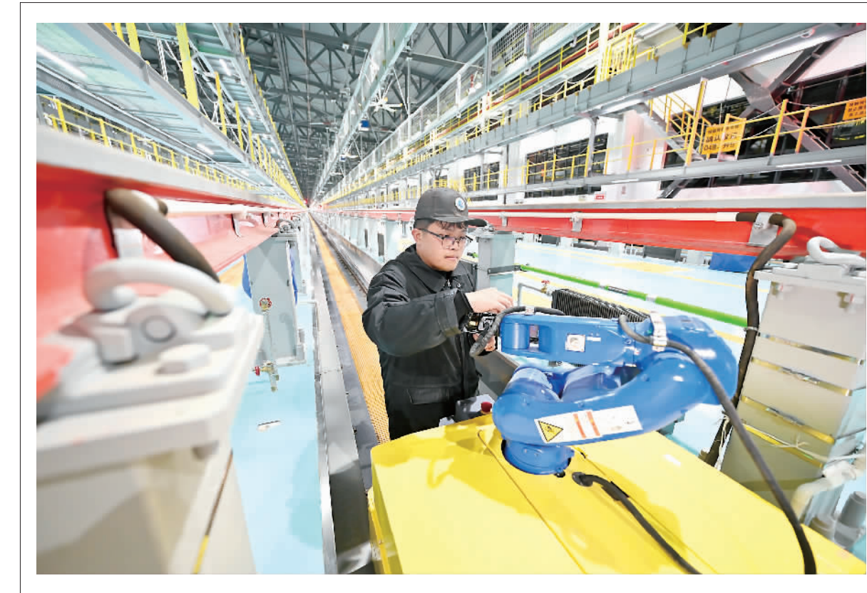
机器人「守护」春运旅途 日前,天津动车客车站利用智能检修机器人对动车组进行一级检修,全力备战春运大考。图为工作人员对智能检修机器人进行作业前状态检查。
